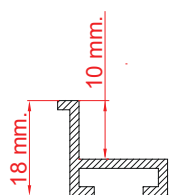
SEZIONE TRASVERSALE TELAIO ALLUMINIO 10 mm
