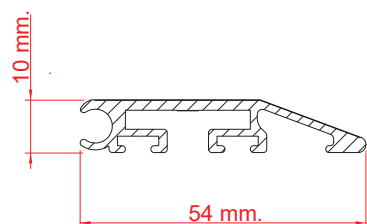
SEZIONE TRASVERSALE RAMPA ALLUMINIO 10 mm
