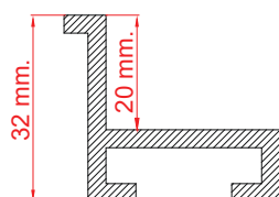
SEZIONE TRASVERSALE TELAIO ALLUMINIO 20 mm
