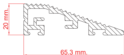
SEZIONE TRASVERSALE RAMPA ALLUMINIO 20 mm
