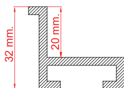
SEZIONE TRASVERSALE TELAIO ALLUMINIO 20 mm
